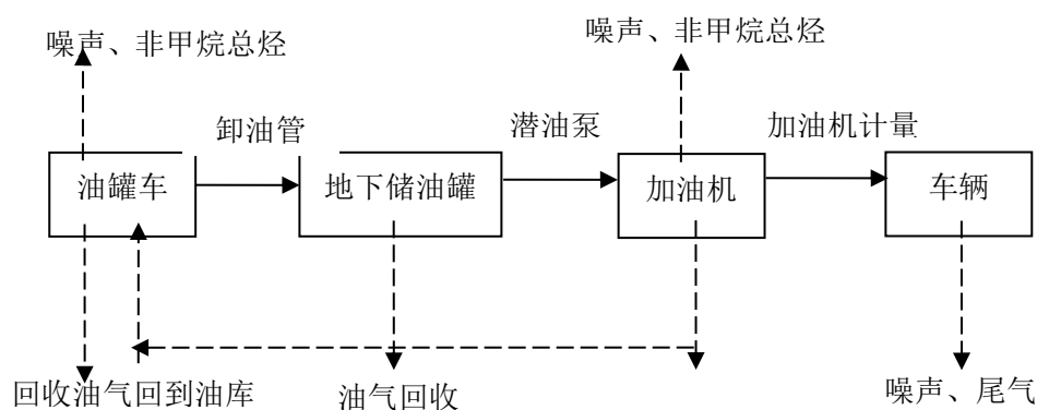
图 2-1 工艺流程图
