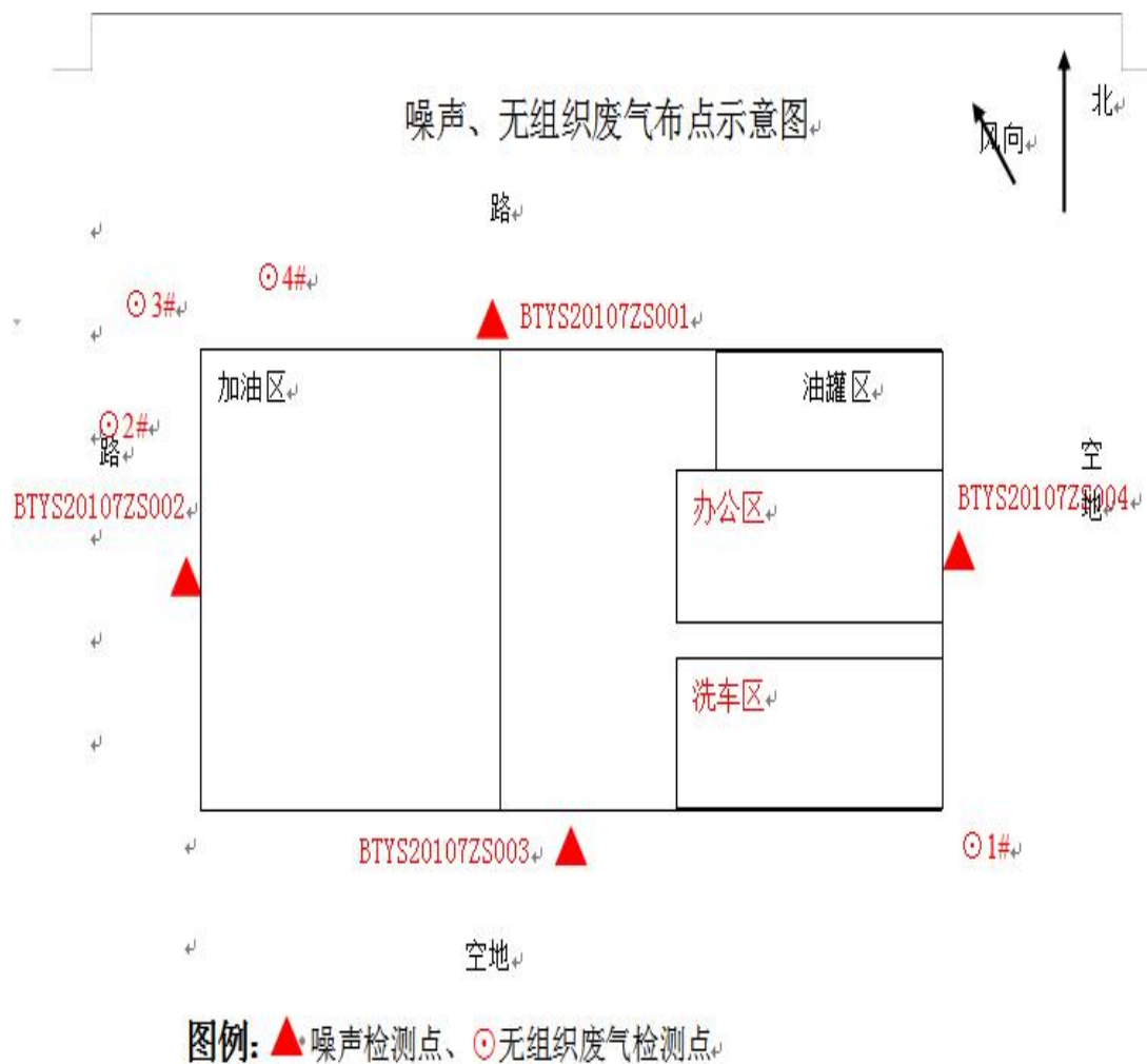
图 6-1 废气及噪声检测点位示意图
