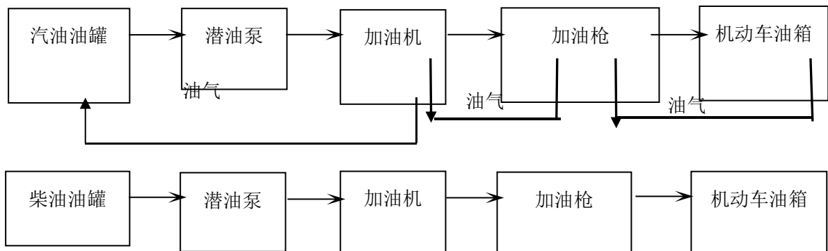
图 2-2 加油工艺流程图
