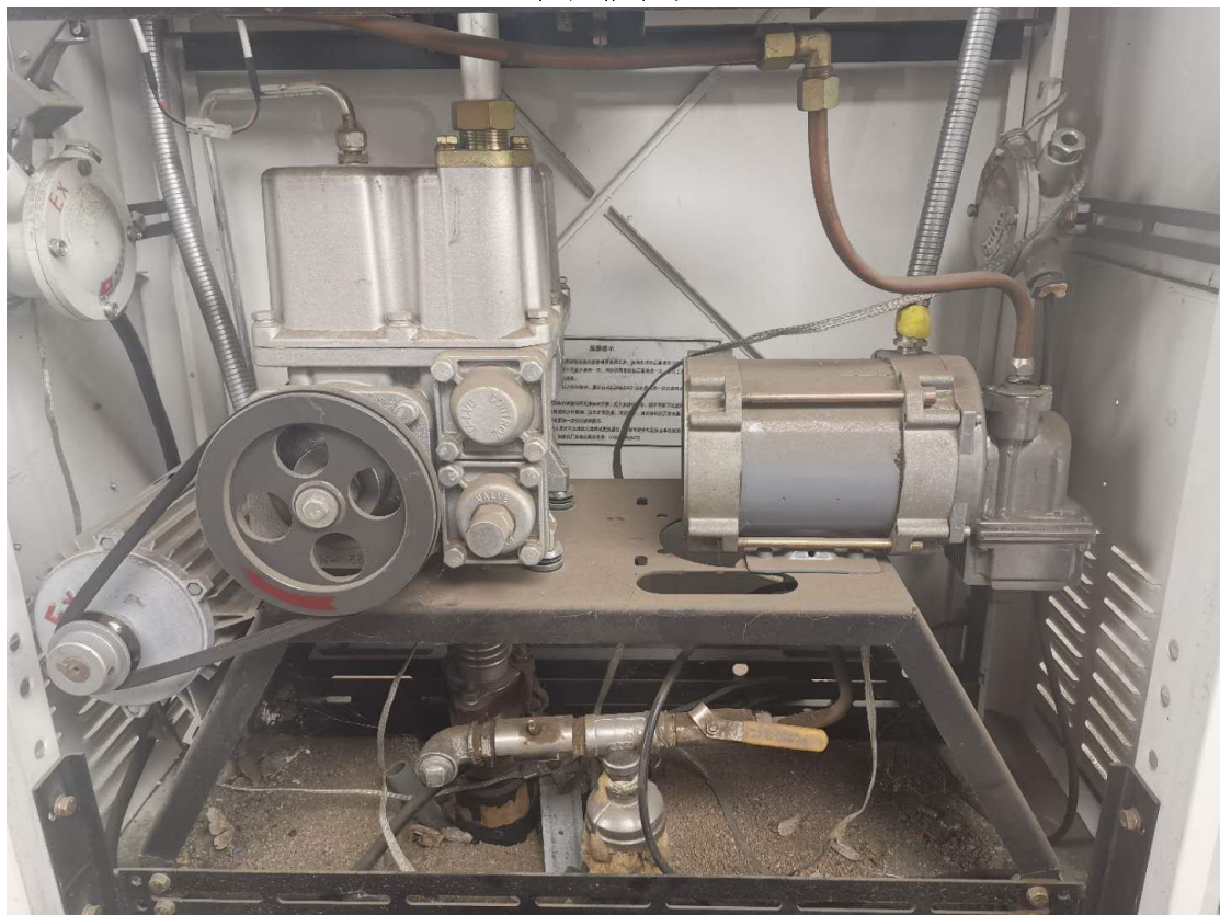
油气回收泵
