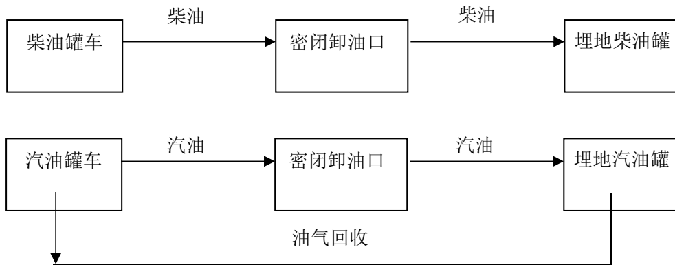
图 2-1 卸油工艺流程图
